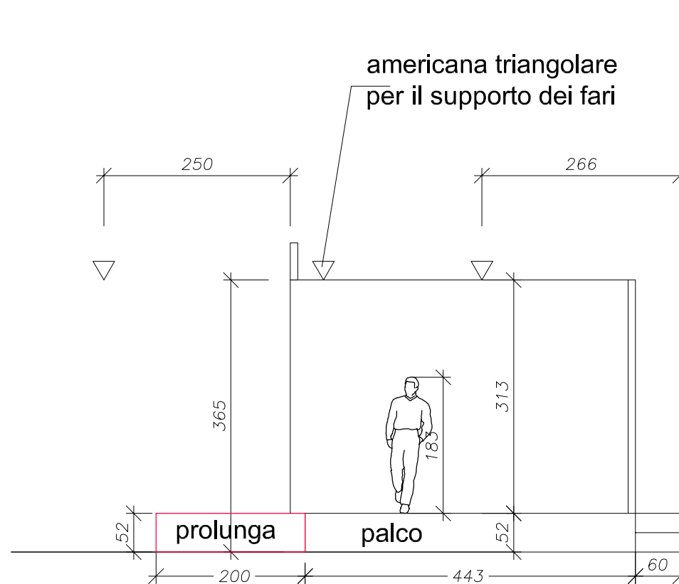
SEZIONE PALCO A-A
